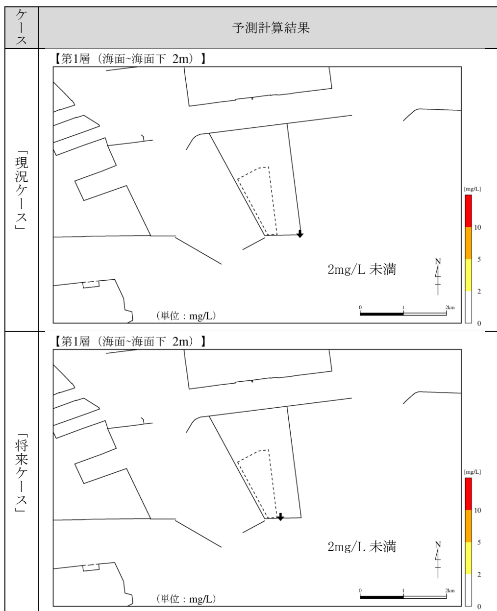
第 11.2.4-28 図 「現況ケース」及び「将来ケース」の予測計算結果 (第 1 層（海面～海面下 2 m）、SS)
