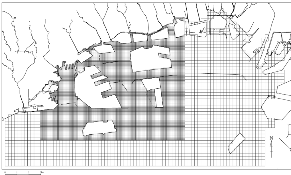
第 11.2.4-8 図（2） 沿岸地形と格子分割（現況地形、中領域）
