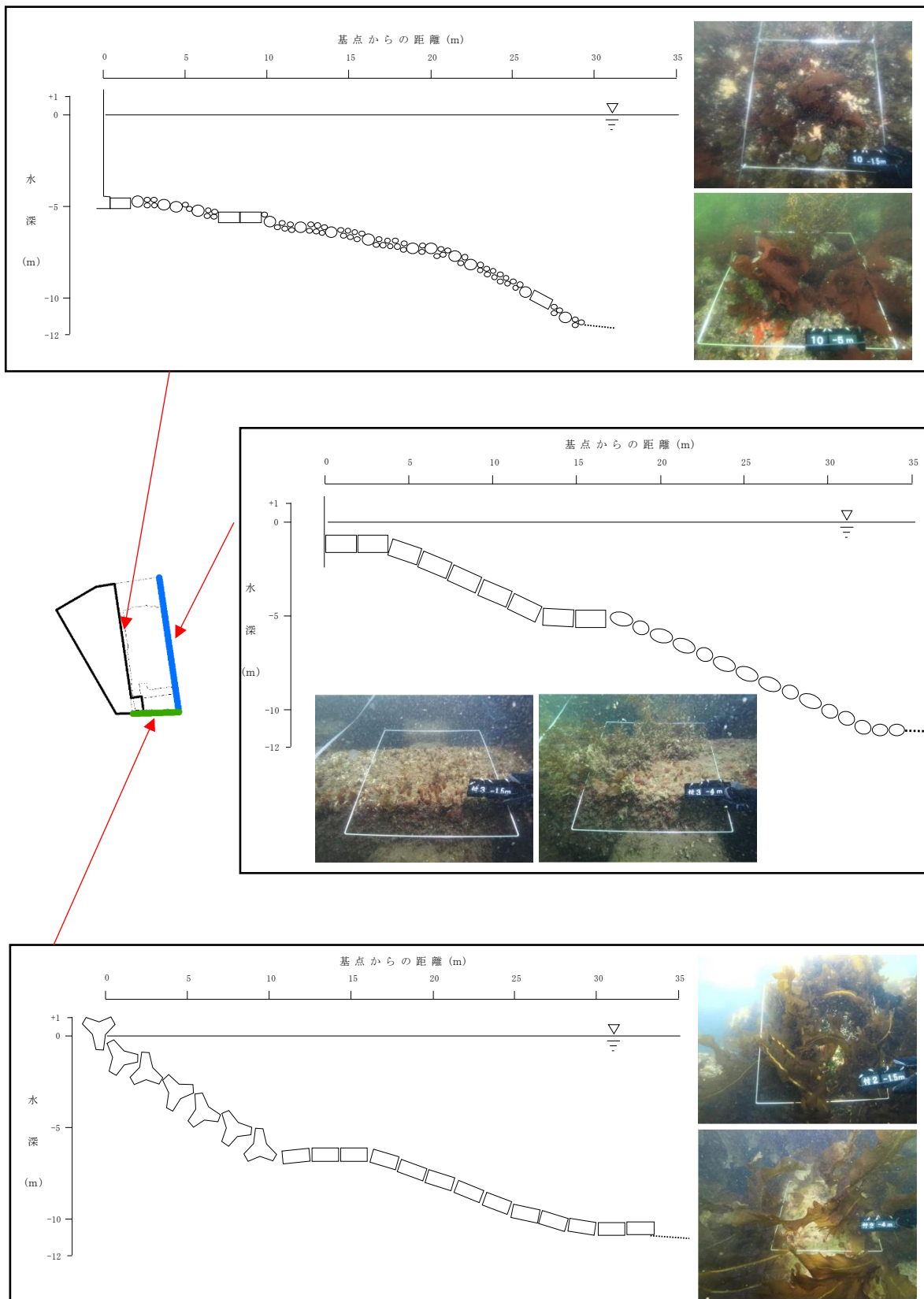
第 11.2.7-3 図 2 期神戸沖埋立処分場周辺の護岸構造及び海藻草類の生育状況
