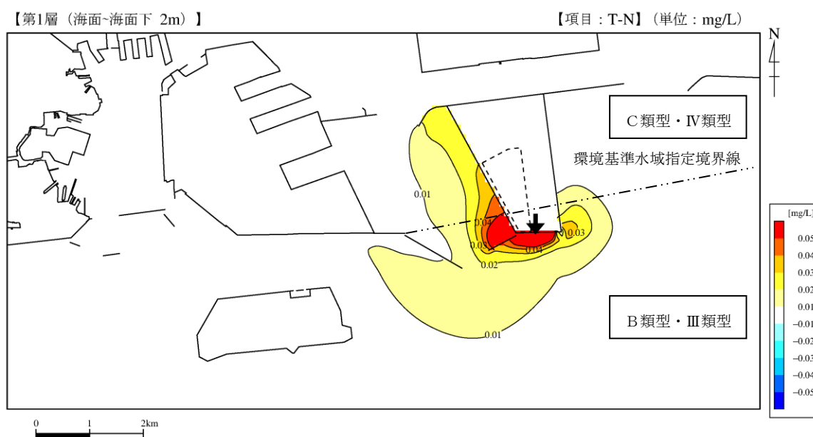
第 11.2.4-24 図（1） 浸出液処理水の排出に伴う水質寄与濃度の予測計算結果 （第 1 層（海面～海面下 2 m）、COD） 【「将来ケース」と「現況ケース」の水質予測結果の差値】
