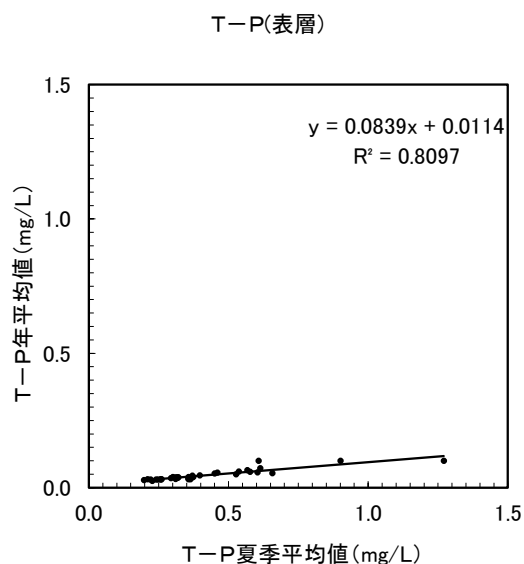
第 11.2.4-26 図 大阪湾における水質の夏季平均値と 75%値または年平均値との関係
