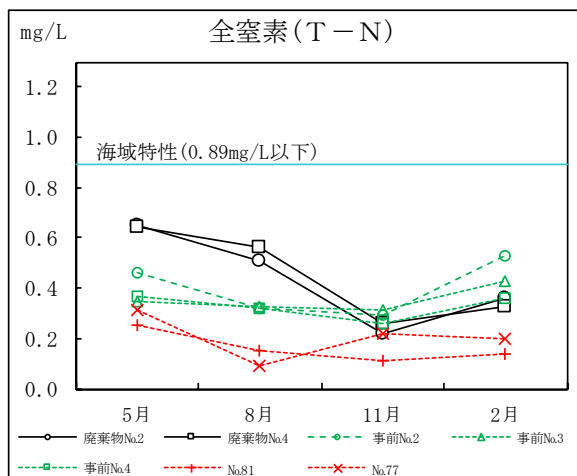
図Ⅱ-3-27 廃棄物受入時の水質の年間推移 (T-N)
