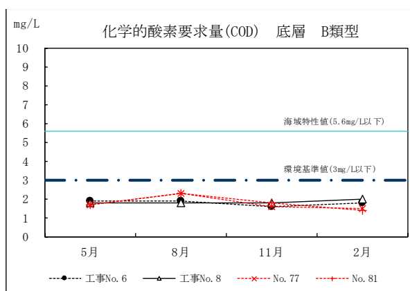
図Ⅱ-3-8 工事中の水質の年間推移 (COD)
