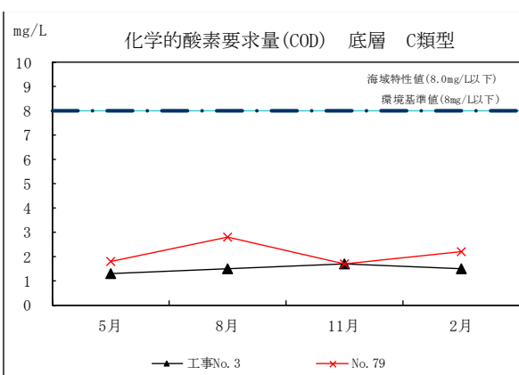
図Ⅱ-3-8 工事中の水質の年間推移 (COD)
