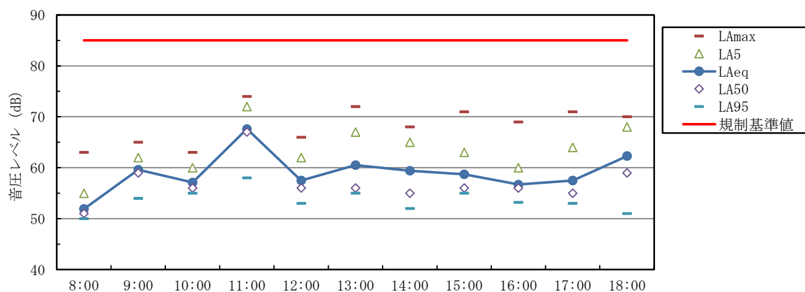
図Ⅱ-2-3 騒音レベルの時間変化（令和2年6月5日）
