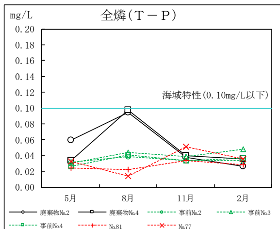
図Ⅱ-3-28 廃棄物受入時の水質の年間推移 (T-P)
