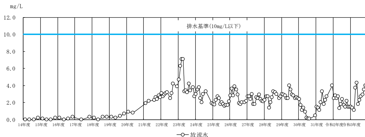
図Ⅱ-3-35 放流水中の溶解性マンガン濃度の経年変化
