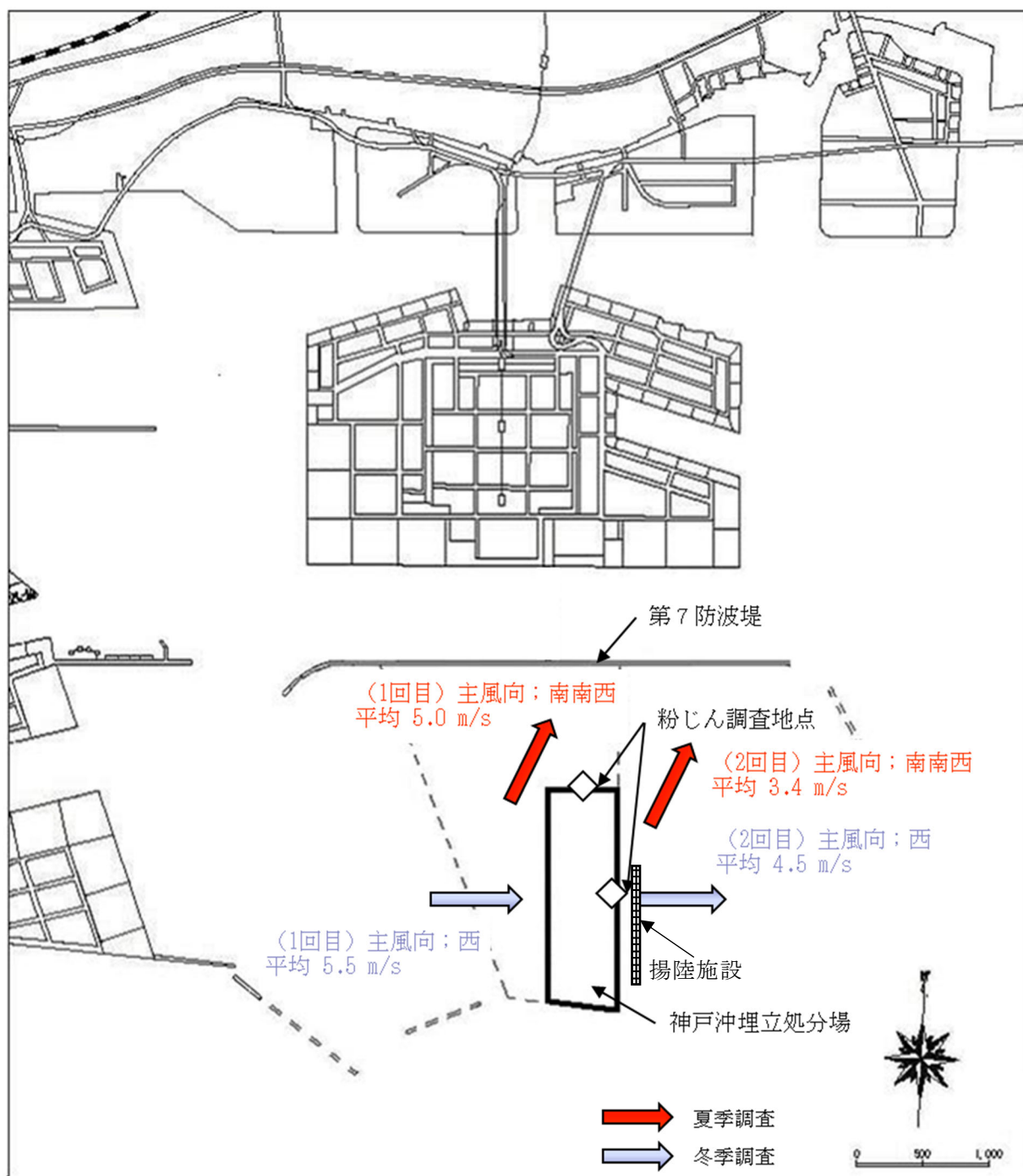
図Ⅱ-1-3 粉じん量調査地点位置図
