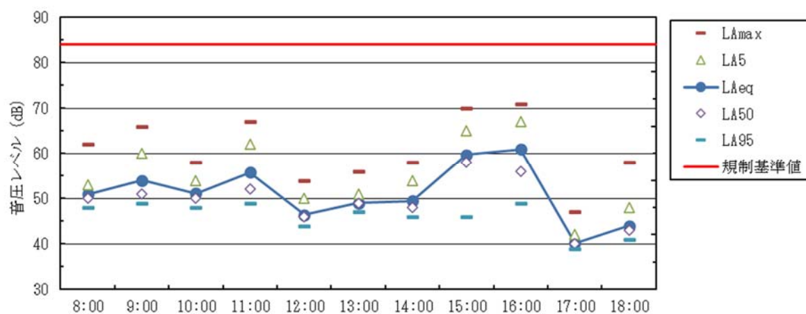
図Ⅱ-2-3 騒音レベルの時間変化（令和3年2月9日）
