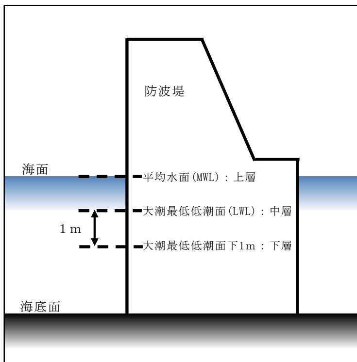
図 II-6-2 模式図
