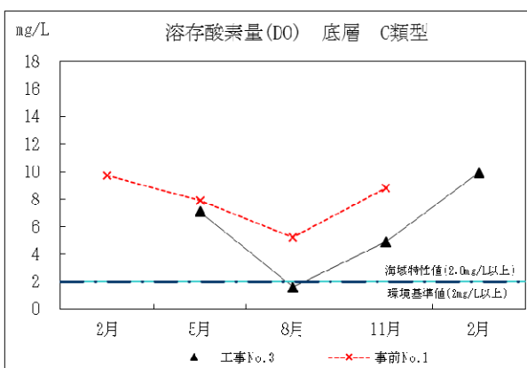
底層
