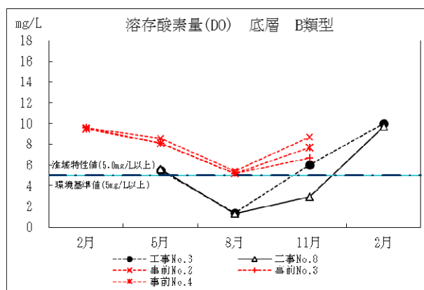
底層
