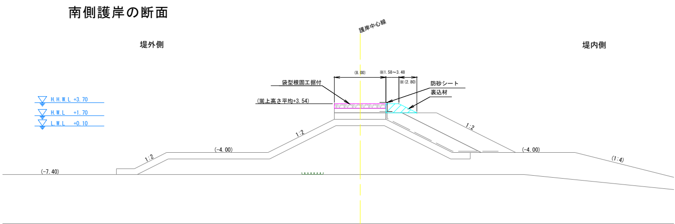
図 I -3-4(2) 潜堤造及び浚渫土による埋立場所の断面図
