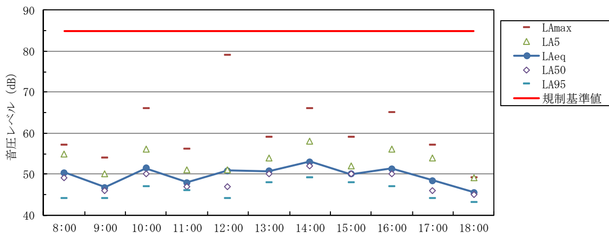
図Ⅱ-2-3 騒音レベルの時間変化（平成30年1月30日：昼間）
