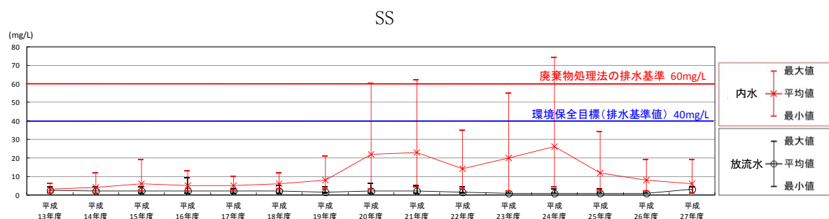
第 3.1.2-4 図 (3)水質調査結果 (廃棄物受入時の内水及び放流水) T-P の推移
