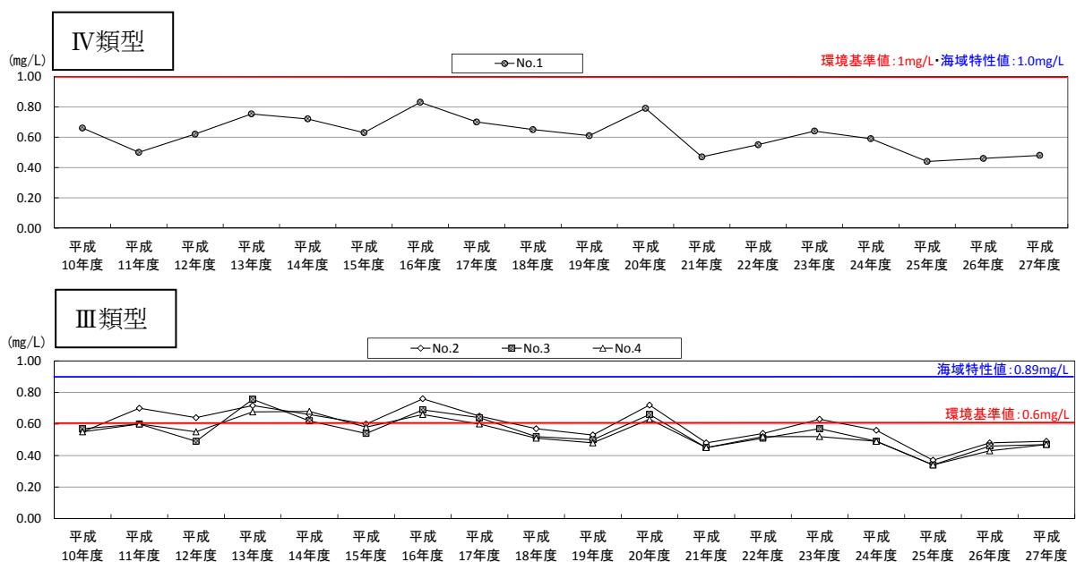
第 3.1.2-3 図 (1)水質調査結果（廃棄物受入時の周辺海域）COD の推移
